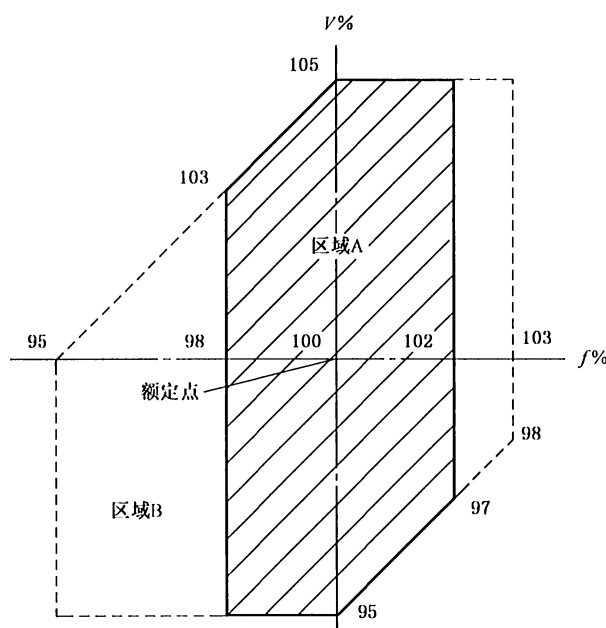
图 1 电压和频率的限值
