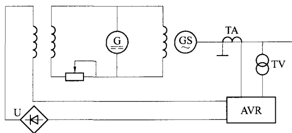
图 15 直流励磁机励磁系统
