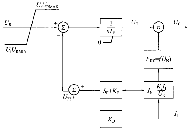
图 14 有励磁变压器的交流励磁机不可控整流器励磁系统功率部分数学模型
