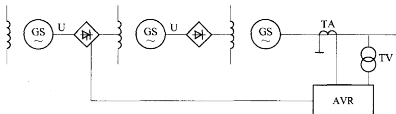
图8 有副励磁机的交流励磁机不可控整流器励磁系统
