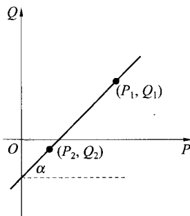
图 B.1 折线型低励限制中的一段直线
