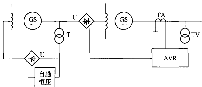
图10 交流励磁机可控整流器励磁系统
