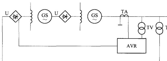
图9 有励磁变压器的交流励磁机不可控整流器励磁系统
