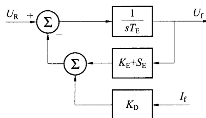
图 16 直流励磁机数学模型
