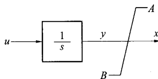
图 A.3 积分环节外限幅
